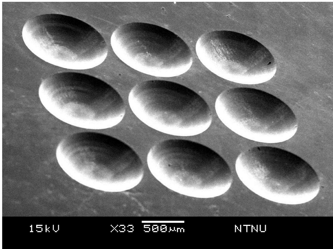
非球面陣列光學微模具
