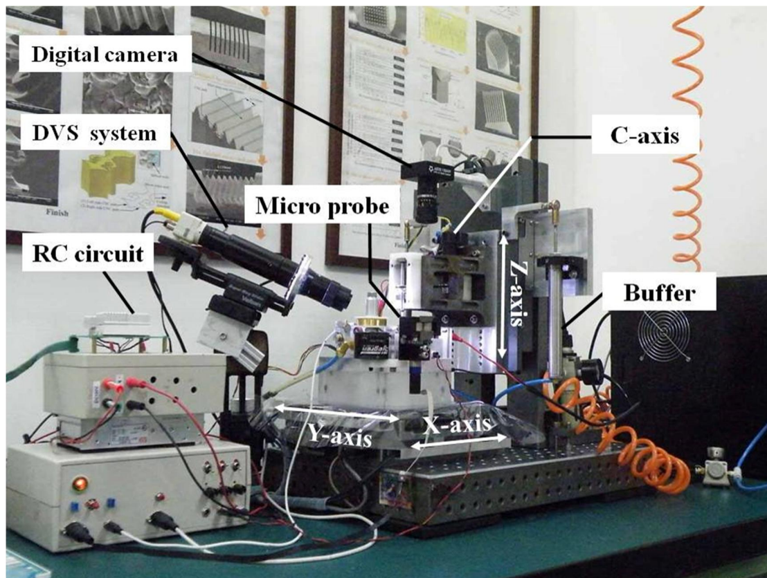
非接觸式精微量測中心機
