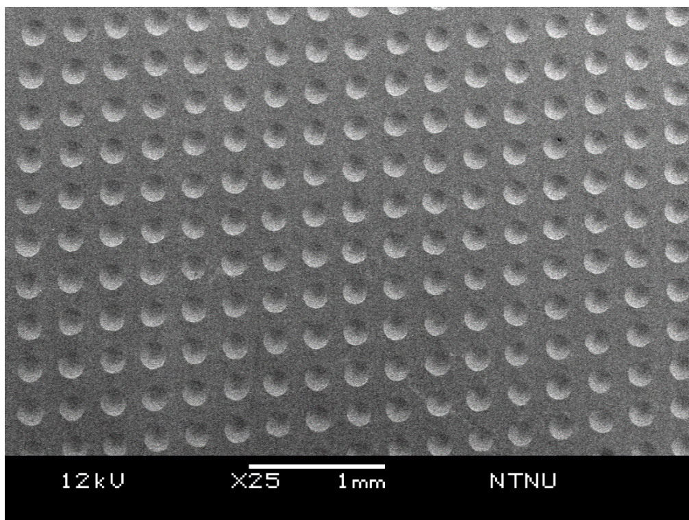
高密度非球面精微模坑陣列
