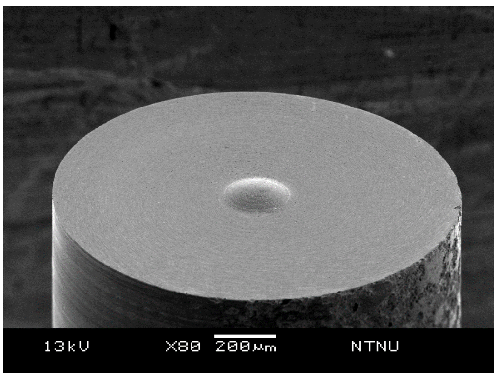
非球面碳化鎢衝擊頭
